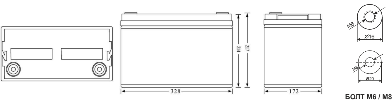
БОЛТ М6 / М8
