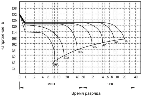
Разрядные характеристики
