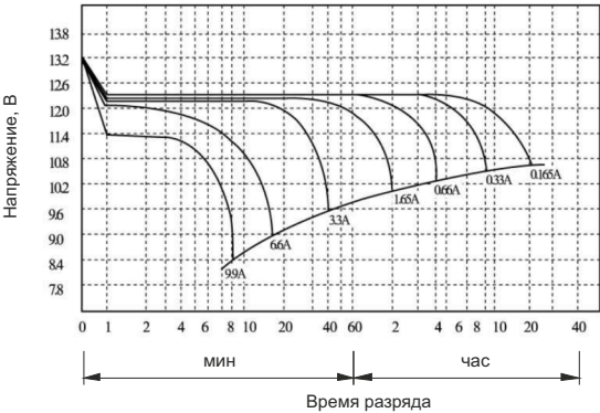
Разрядные характеристики
