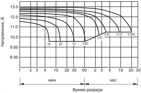
Разрядные характеристики
