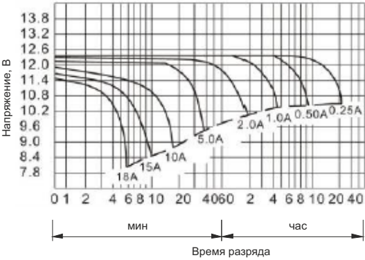
Разрядные характеристики
