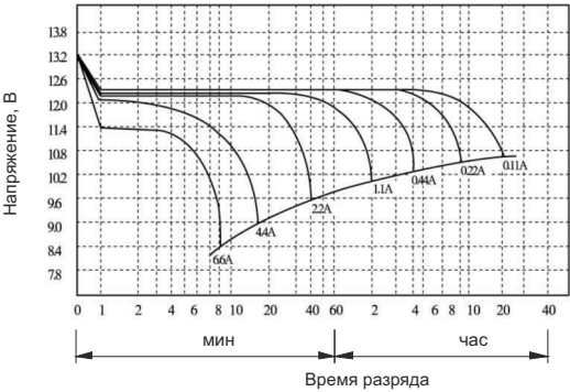
Разрядные характеристики
