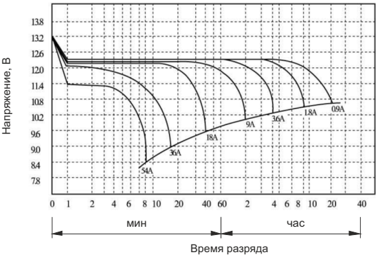
Разрядные характеристики
