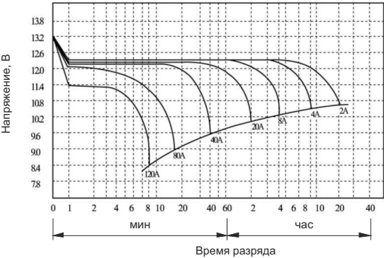
Разрядные характеристики
