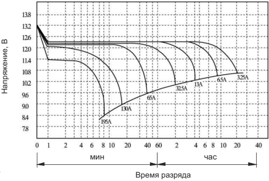
Разрядные характеристики
